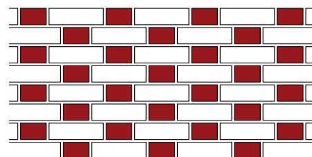
Фламандская
